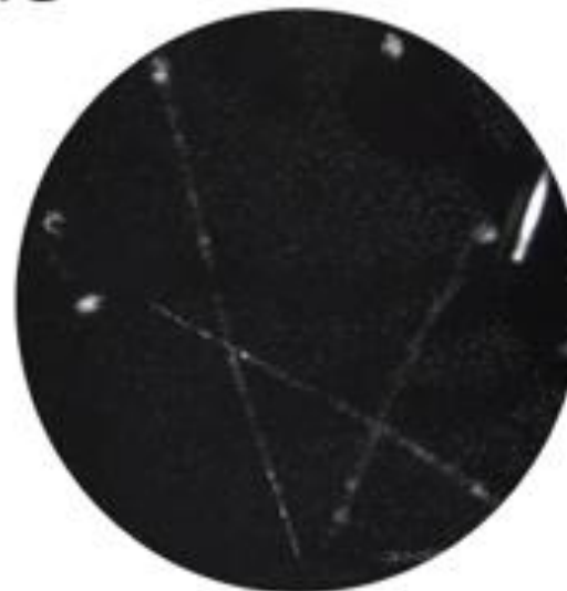
Muons
